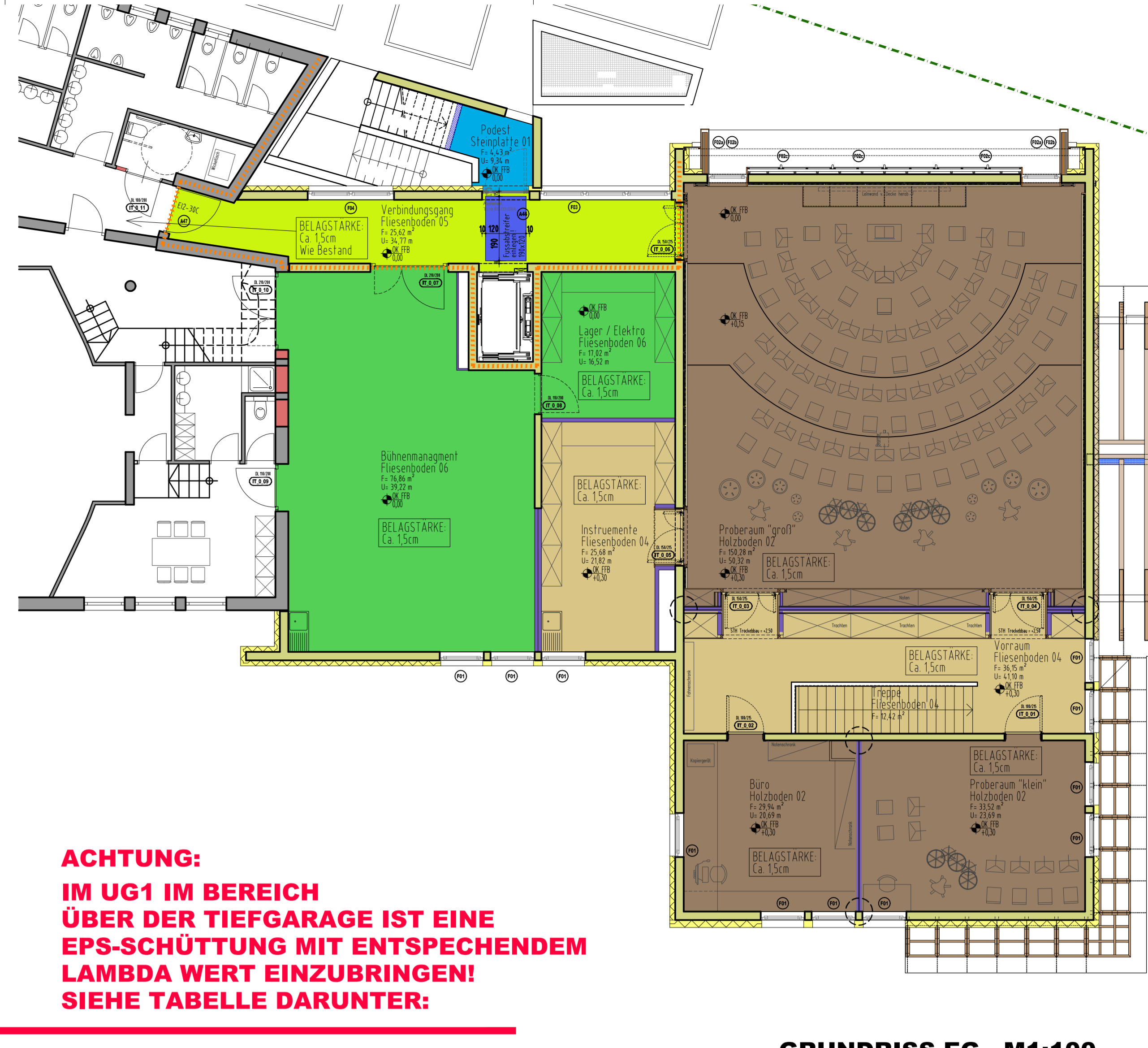
GRUNDRISS EG M1:100
