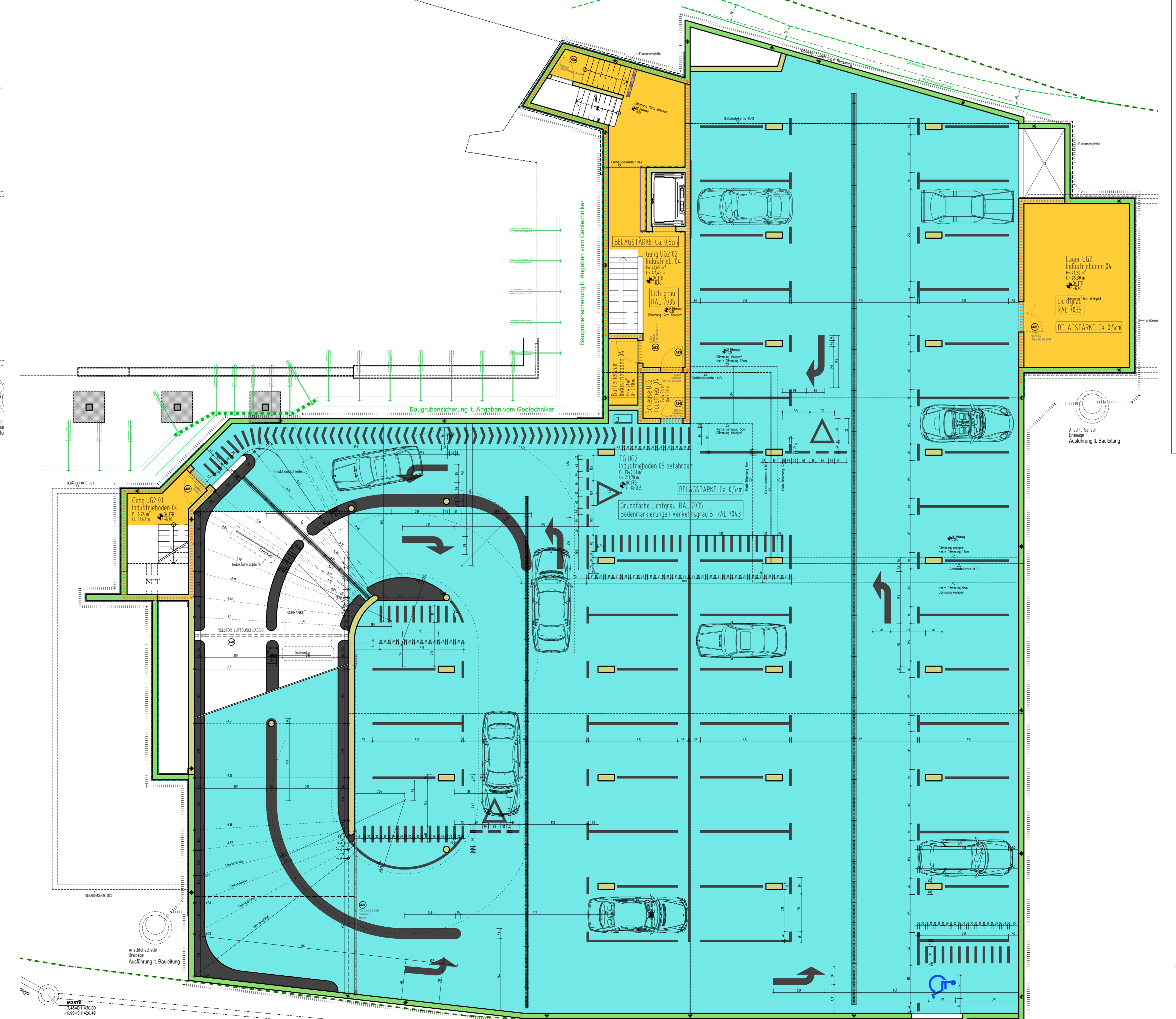
GRUNDRISS UG2 M1:100
